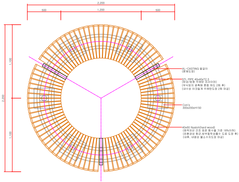
1 정면도 SCALE=A1 : 1/10 A3 : 1/20
