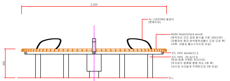
2 정면도 SCALE=A1 : 1/10 A3 : 1/20
